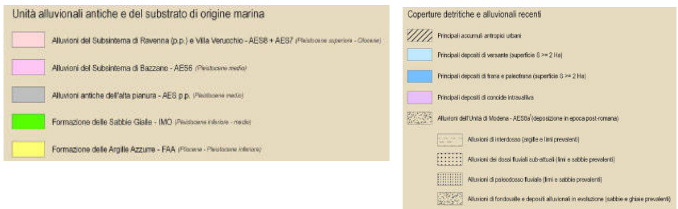
Fig. 1: Estratto della Carta geologica del PSC associato (Quadro conoscitivo).
